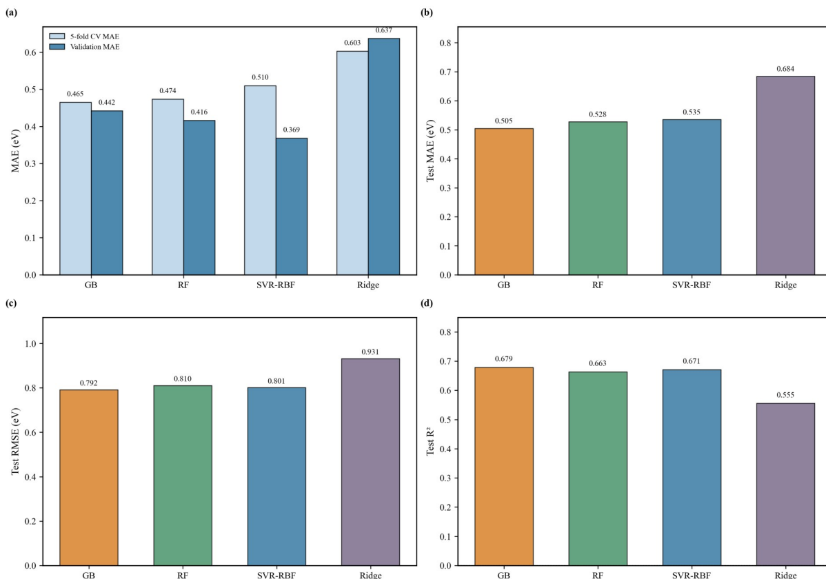
图 6 基线模型性能比较
