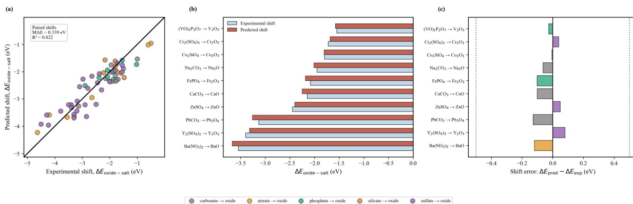
图 11 盐/氧化物配对体系的 O 1s 相对位移预测
