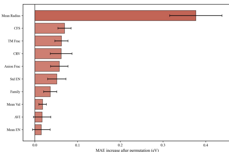
图 10 增强模型的置换特征重要性
