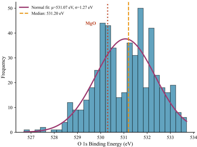
图 1 数据库中 O 1s 结合能分布
