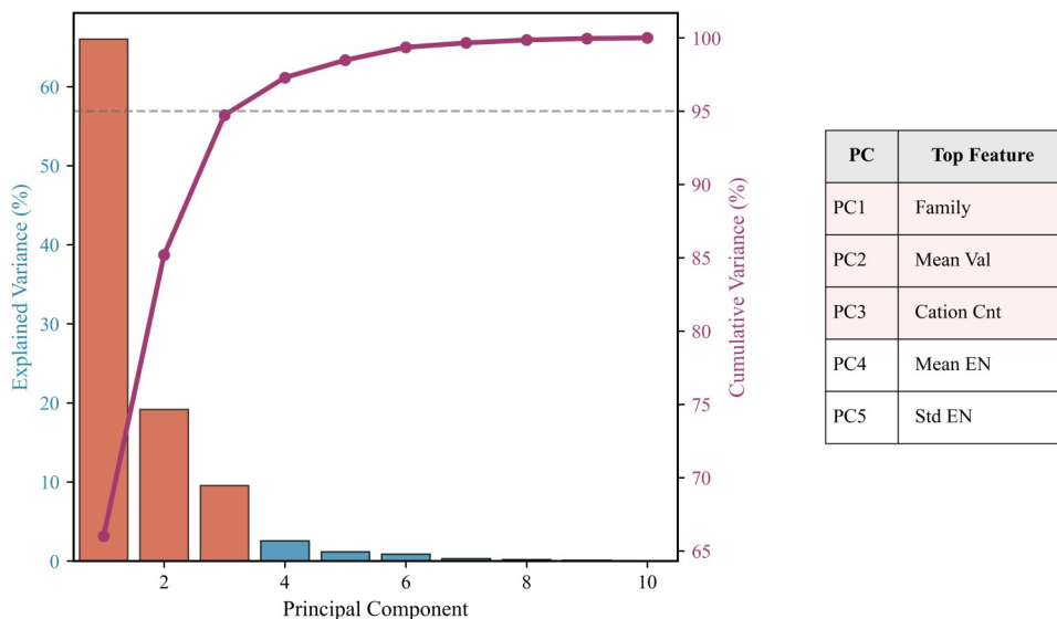
图3 基线组成描述符的主成分分析
